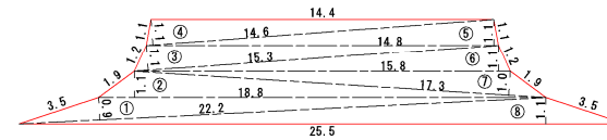
車道取付け舗装展開図
