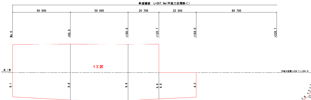
車道取付け舗装展開図
